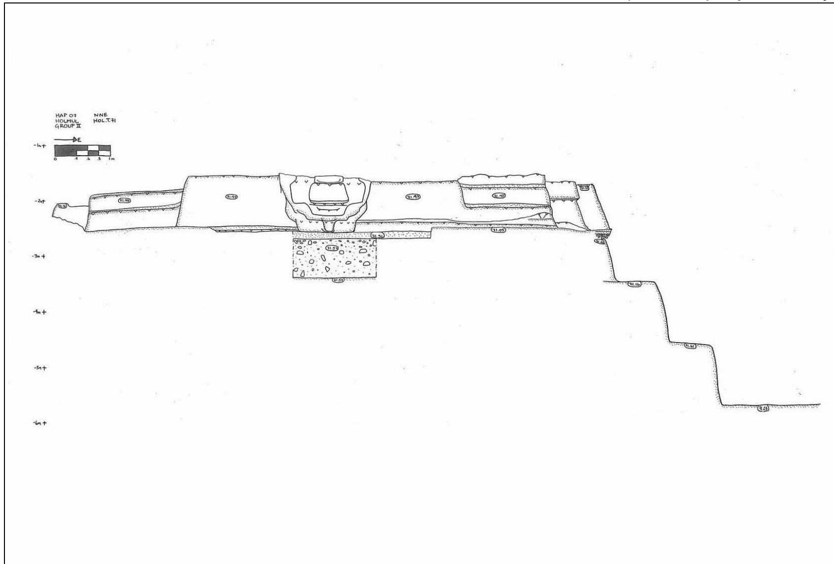
Figura 6. Perfil E-0 de la fachada sur del Edificio N.
